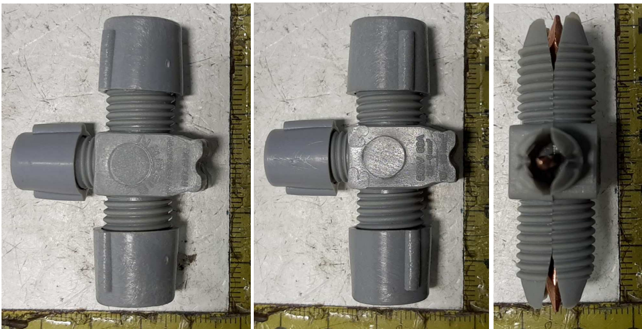
Vistas del conector para empalmes y derivaciones
