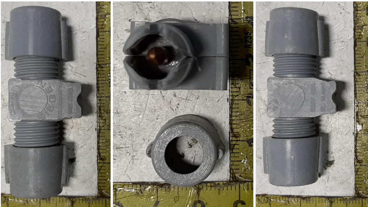
Vistas del conector para empalmes
